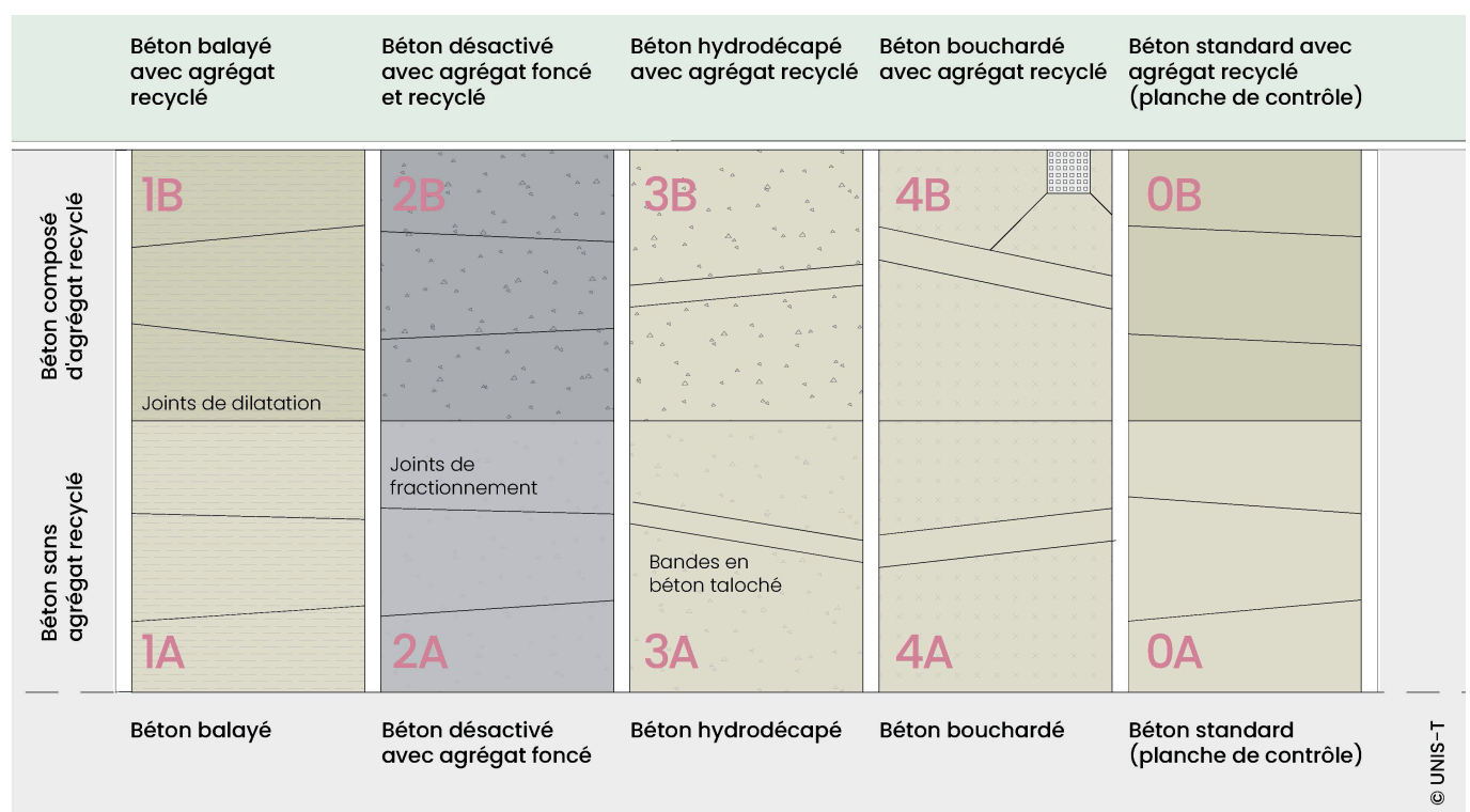
Plan d'installation des planches d'essai avec détails des différentes compositions et des traitements de surface
